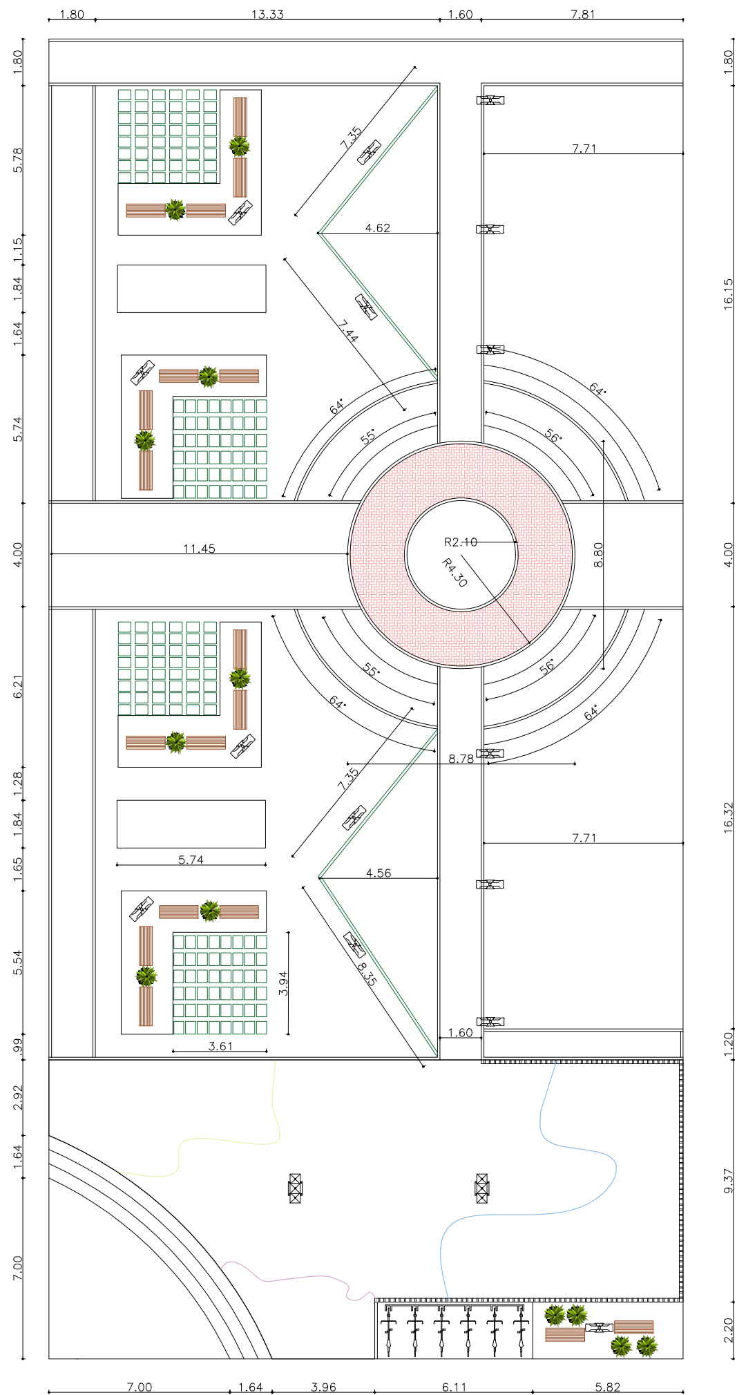
PLANTA BAIXA esc 1:100
